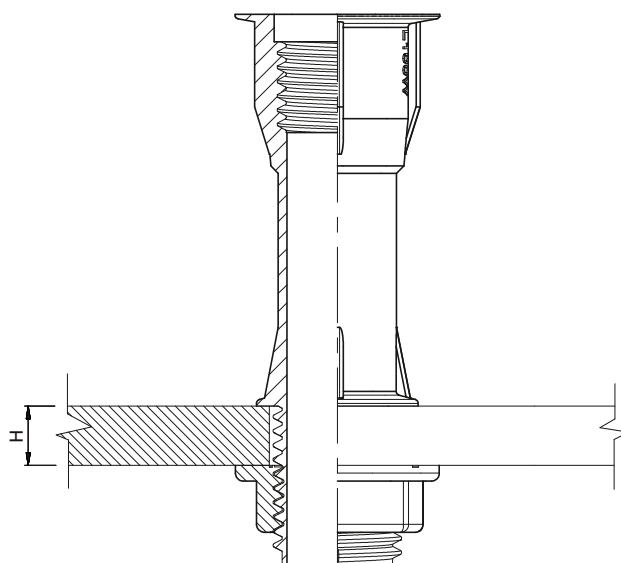
МОНТАЖ НА ПЛОЧА / MOUNTING ON PLATE
